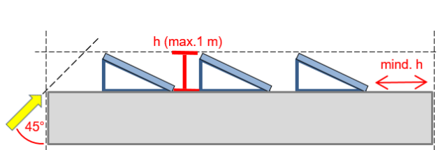
Abb. 5: 1 m-Regel und Einrückung, mindestens im Umfang der Aufständerungs-Höhe
