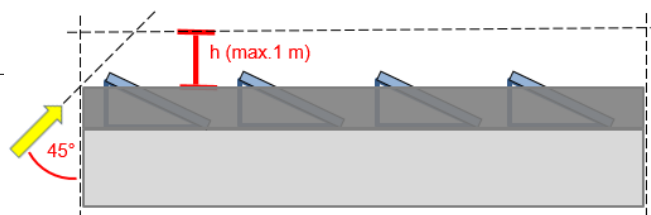
Abb. 6: 1 m-Regel und Einrückung bei Vorliegen einer undurchsichtigen (opaken) Brüstung
