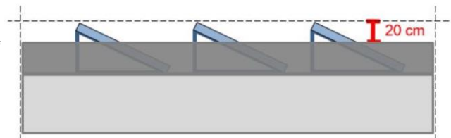
Abb. 4: Abstand von 20 cm ab undurchsichtiger (opaker) Brüstung
