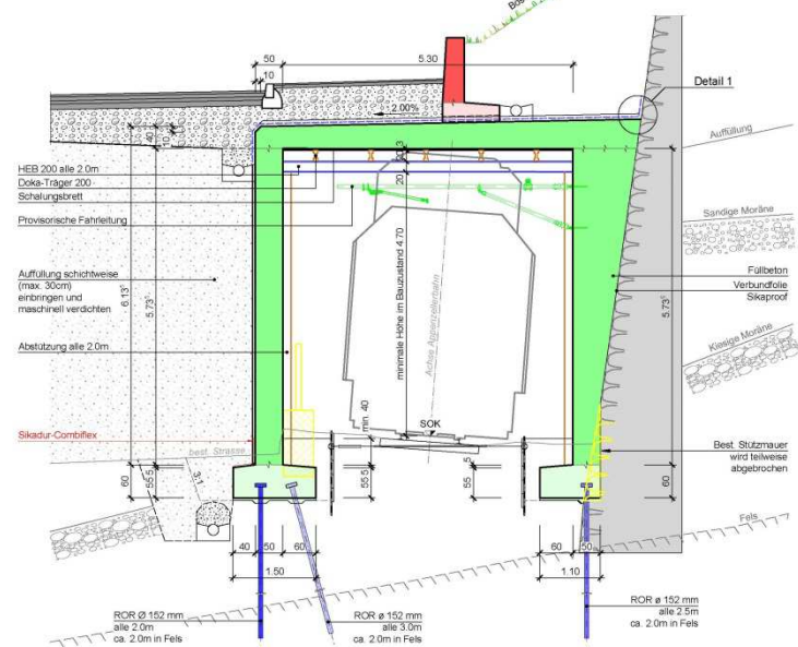
Schnitt B - B 1:50 Bauzustand
