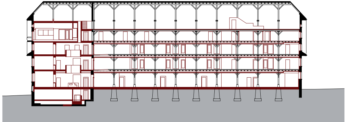
Längsschnitt Zeughaus
