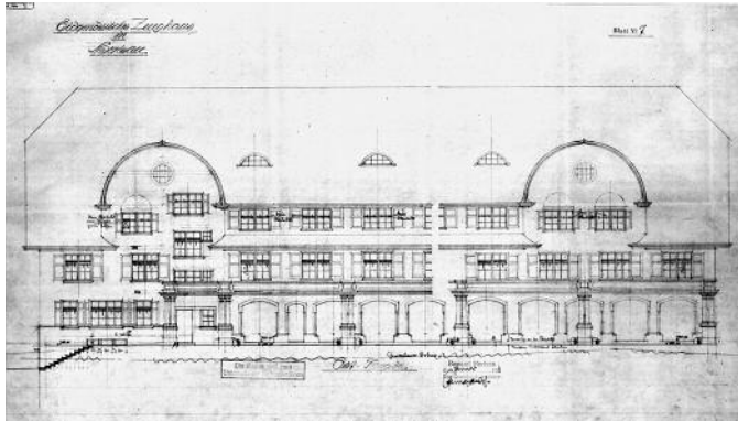
Ramseyers Ausführungsplan vom Januar 1918 (Hochbauamt AR)
