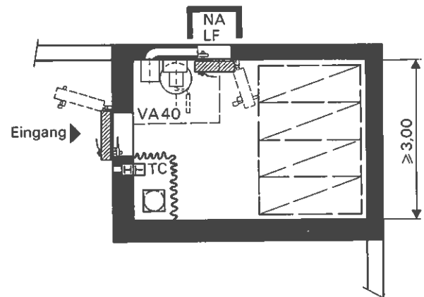
Figur 2.4-6 Grundrissform für 12 Schutzplätze (Bodenfläche \geq 13 m 2 )
