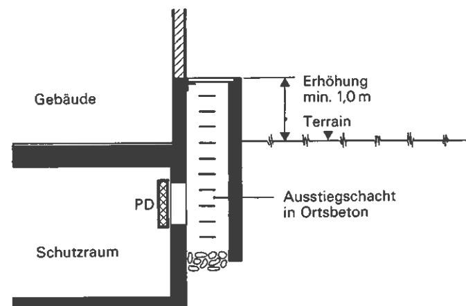
Figur 2.3-2 Notausstieg mit erhöhtem Ausstiegsschacht
