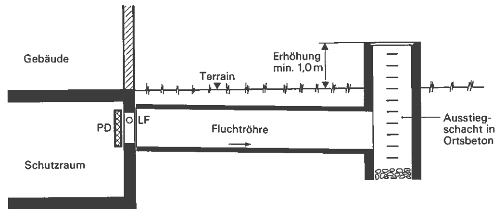
Figur 2.3-1 Fluchtröhre mit erhöhtem Ausstiegsschacht
