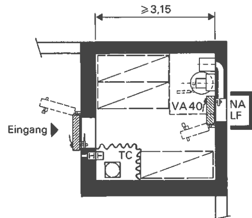
Figur 2.4-4 Grundrissform für 9 Schutzplätze (Bodenfläche \geq 10 m 2 )
