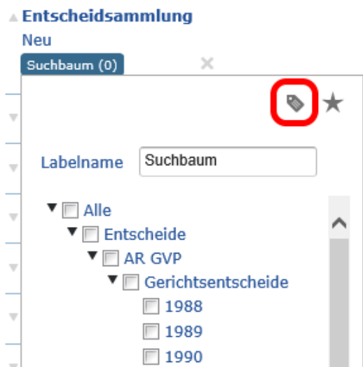
Abbildung 3: Suchbaum
